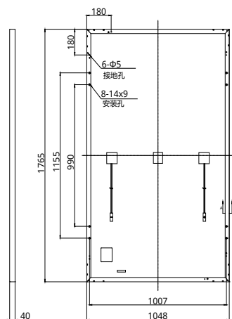
背面图
