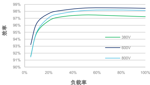
效率曲线
