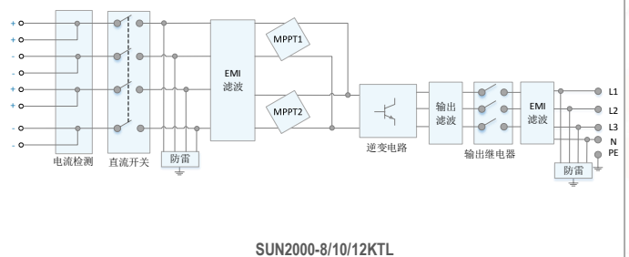
电路框图
