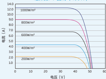
组件的I-V曲线(490W)
