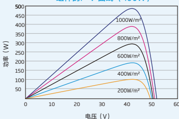
组件的P-V曲线(490W)
